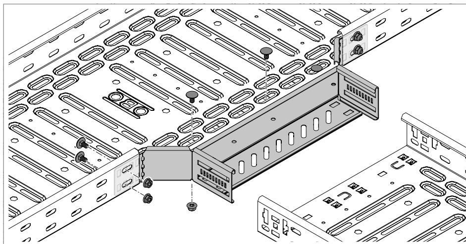
Figura 56: Aparafusar a derivação simples ao caminho de cabos em chapa contínua
