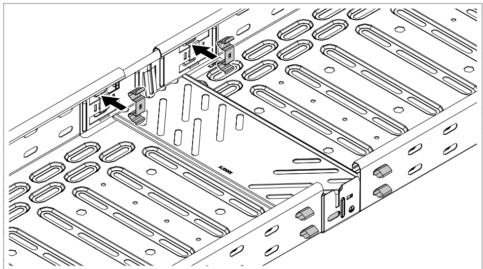
Figura 24: Fixar a união com grampos duplos
