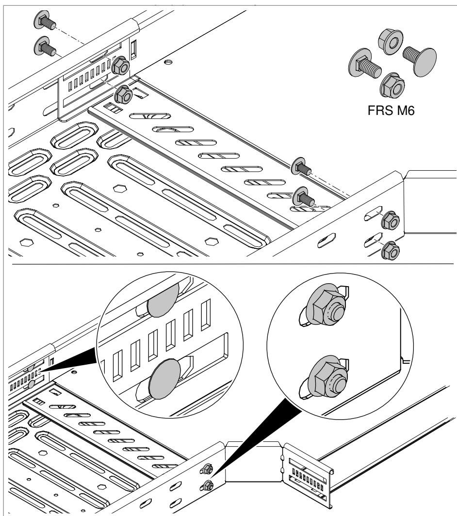
Figura 52: Fixar o acessório com grampos duplos
