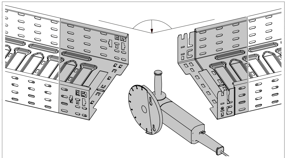
Figura 29: Cortar o caminho de cabos em chapa para criar ângulos
