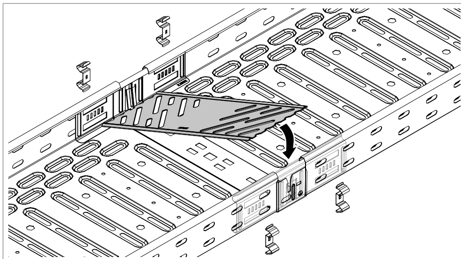
Figura 22: Introduzir a régua tapa juntas da união reta KTSM
