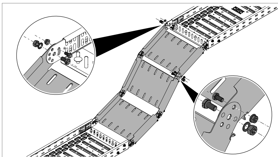
Figura 71: Montar elementos do ângulo regulável
