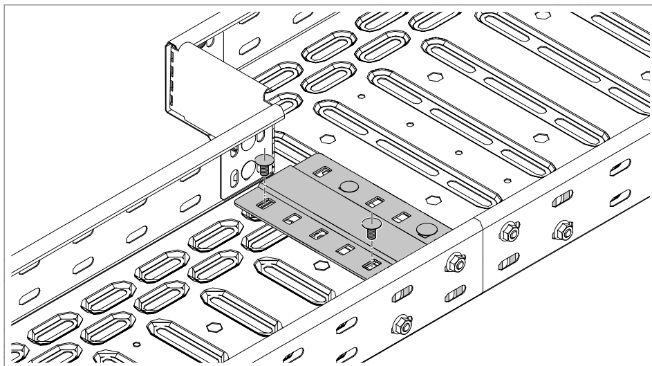
Figura 74: Aparafusar a régua tapa juntas
