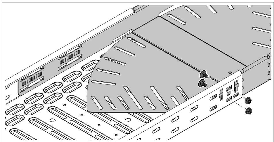
Figura 60: Fixar o ângulo variável
