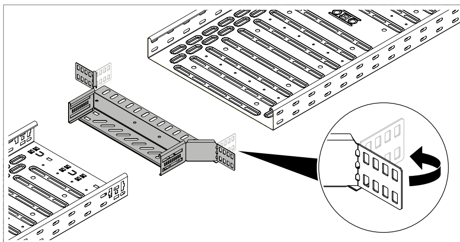
Figura 57: Dobrar a patilha de ligação
