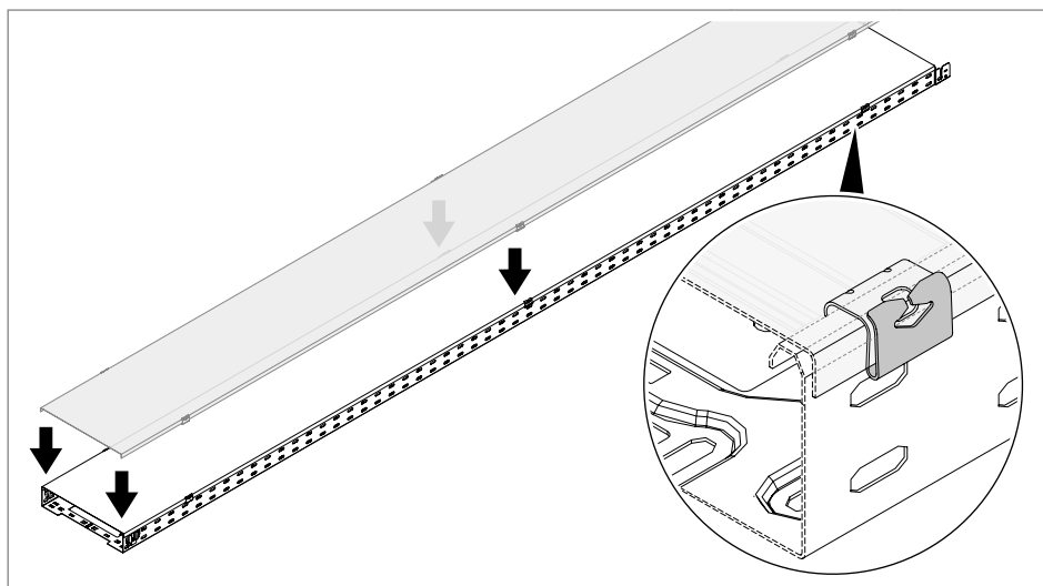
Figura 84: Encaixar a tampa
