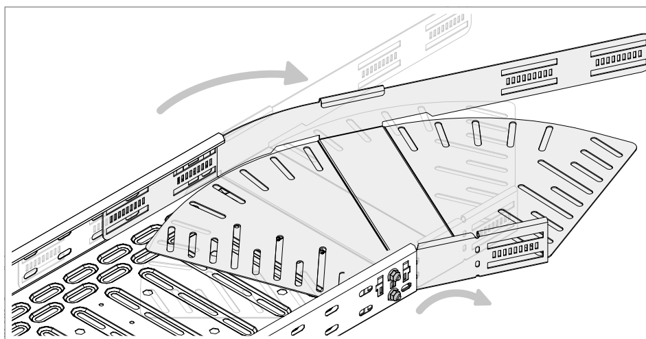
Figura 61: Dobrar o ângulo variável
