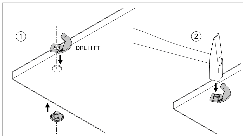
Figura 87: Rebitar o ferrolho
