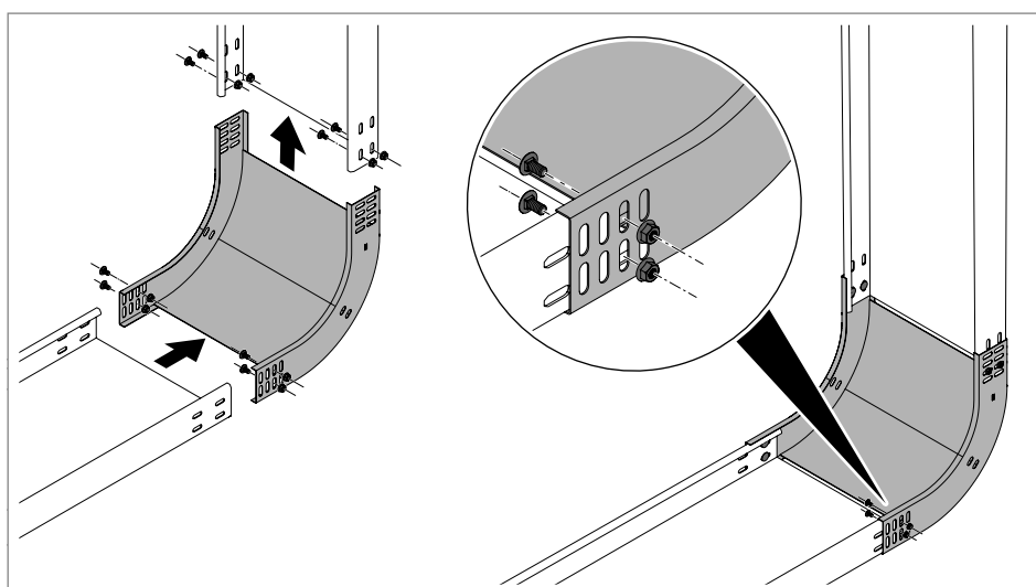
Figura 67: Montar ângulo vertical de subida
