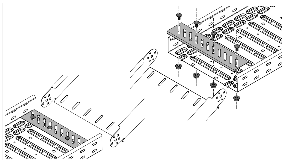
Figura 69: Montar a placa de fundo
