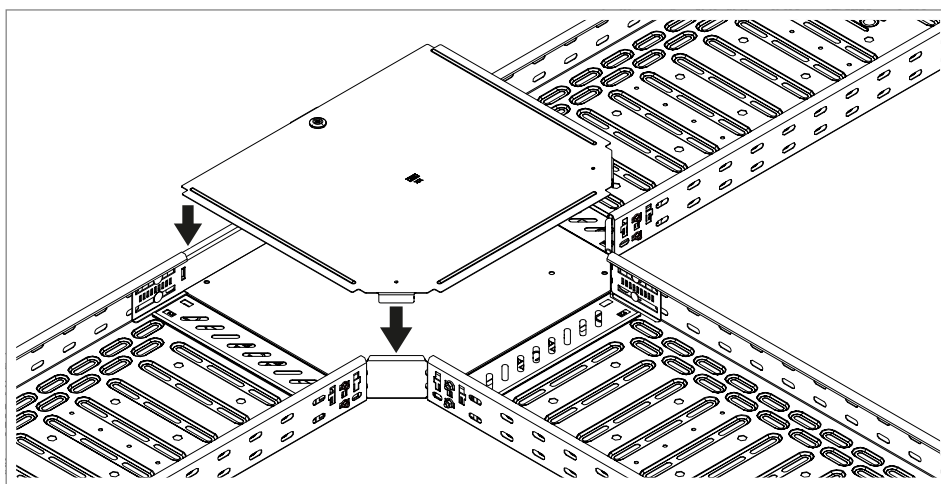
Figura 89: Colocar a tampa do acessório
