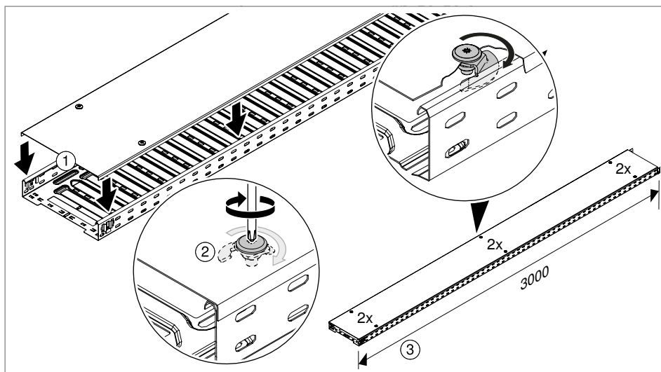
Figura 88: Montar a tampa com ferrolho de hélice
