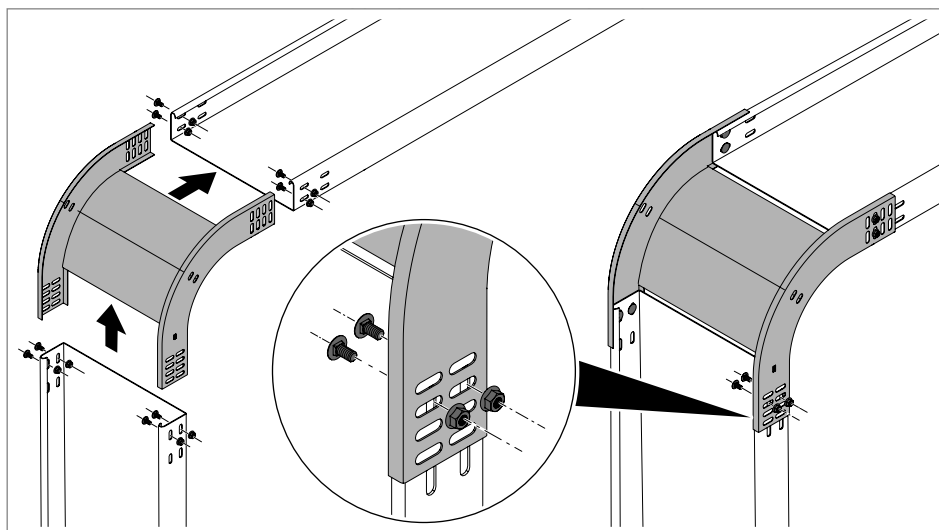
Figura 66: Montar ângulo vertical de descida
