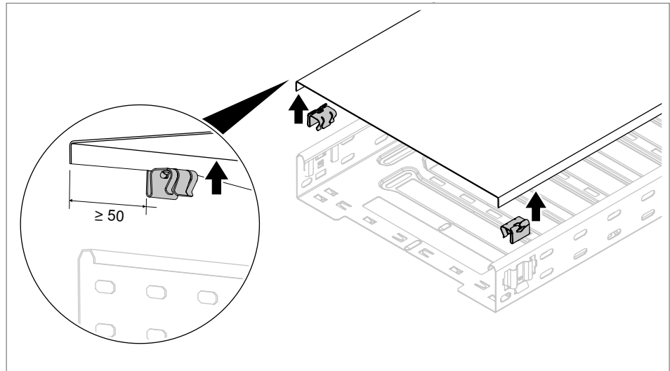
Figura 82: Prender o grampo na tampa
