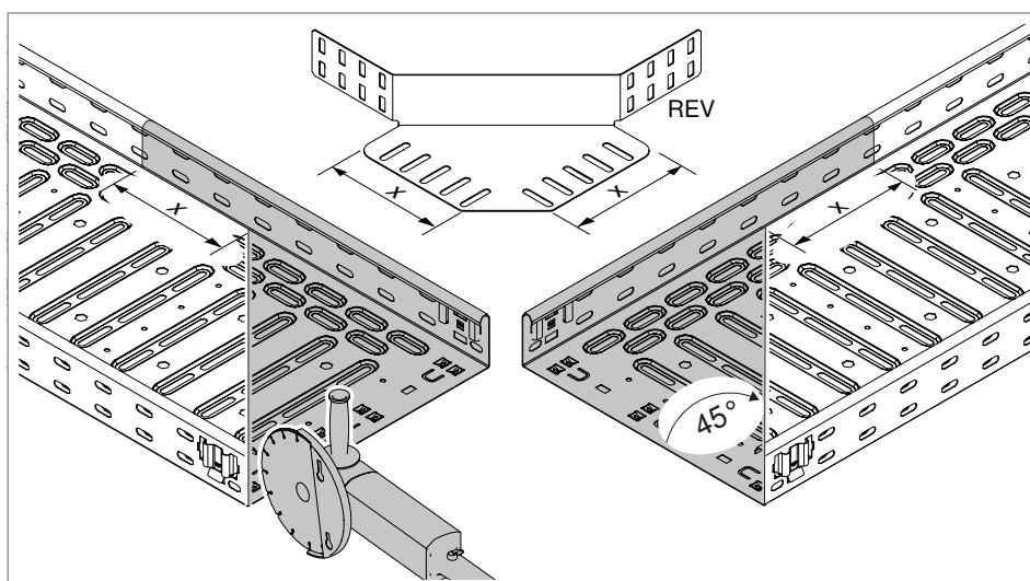
Figura 35: Cortar caminhos de cabos em chapa para o conector de canto REV
