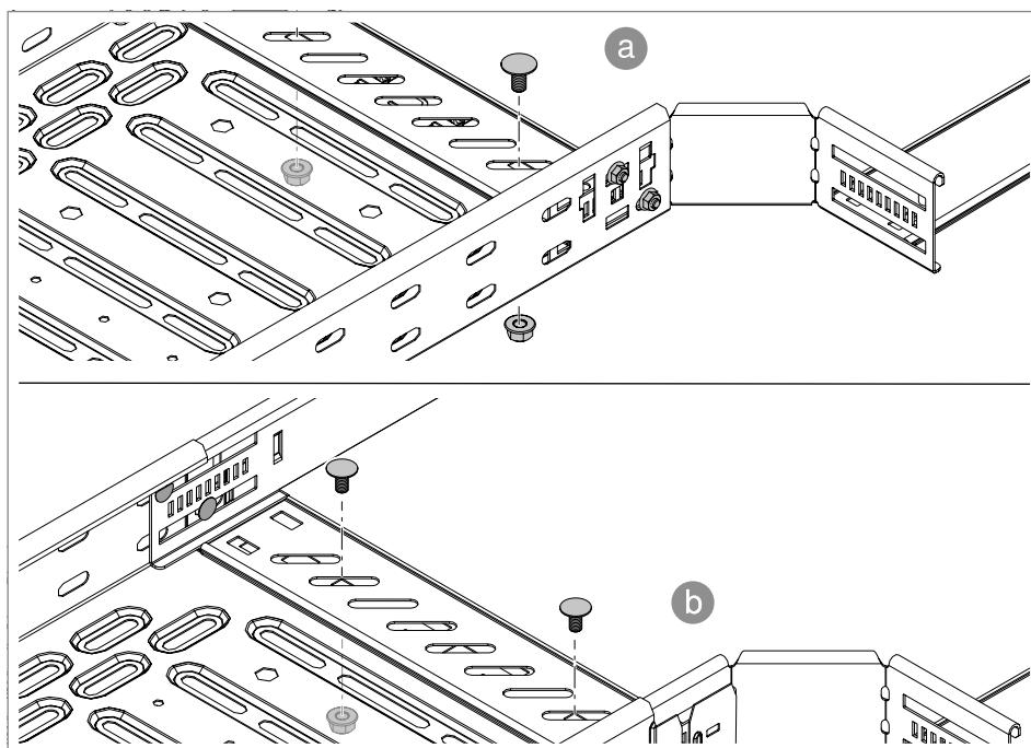
Figura 49: Aparafusar a régua tapa juntas (extremidade do caminho de cabos a e b )
