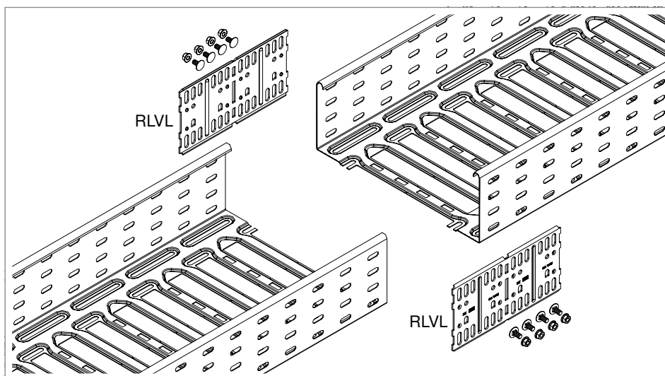
Figura 26: Uniões retas e curvas RLVL
