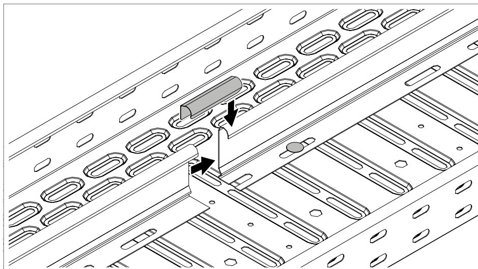
Figura 80: Unir os separadores
