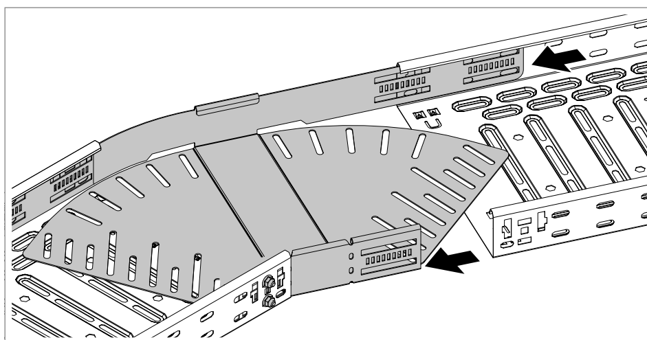
Figura 62: Inserir o segundo caminho de cabos no ângulo
