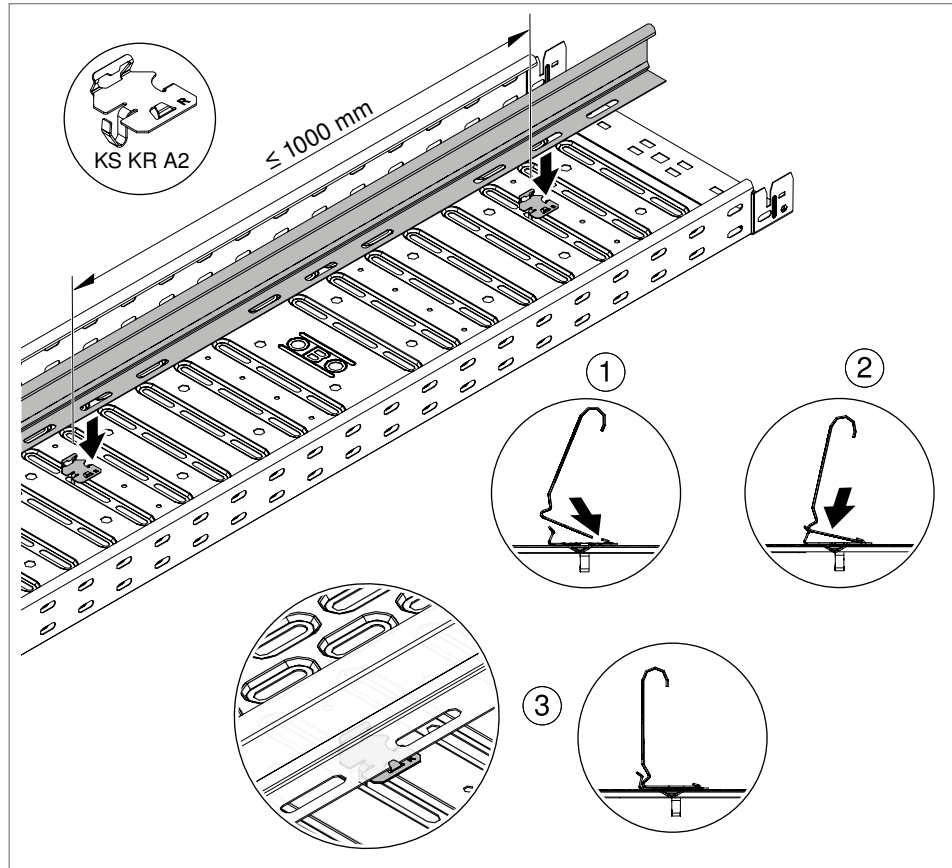
Figura 79: Inserir o separador no fixador
