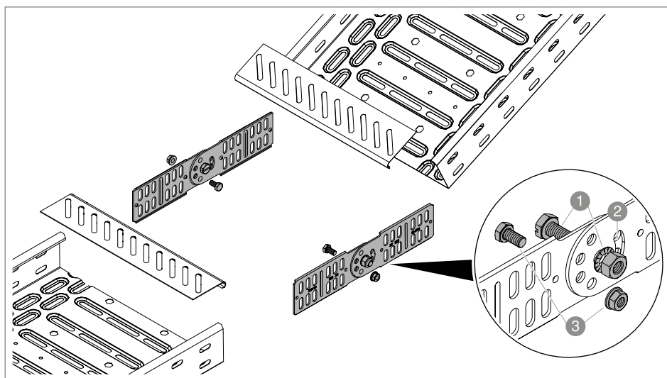
Figura 37: Uniões articuladas RGV e placas de fundo
