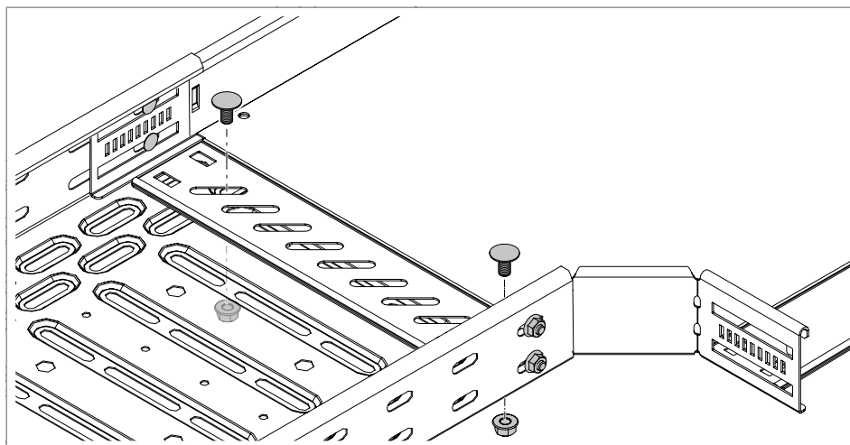
Figura 53: Aparafusar a régua tapa juntas
