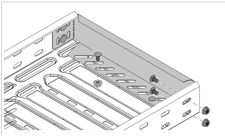
Figura 76: Montar o topo
