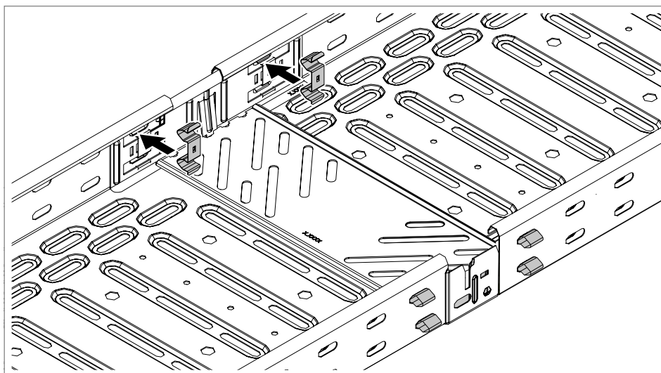
Figura 23: Fixar a união com grampos duplos
