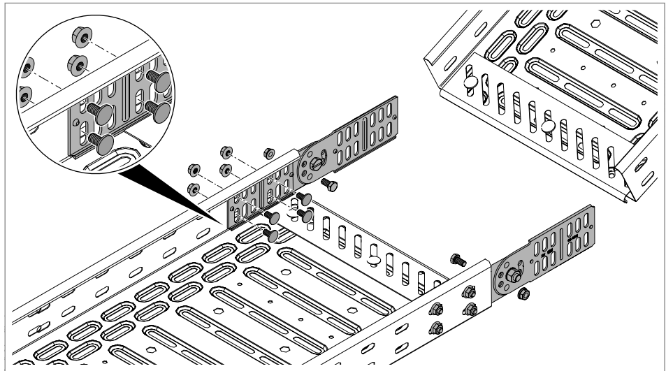
Figura 39: Aparafusar as uniões articuladas RGV ao caminho de cabos em chapa
