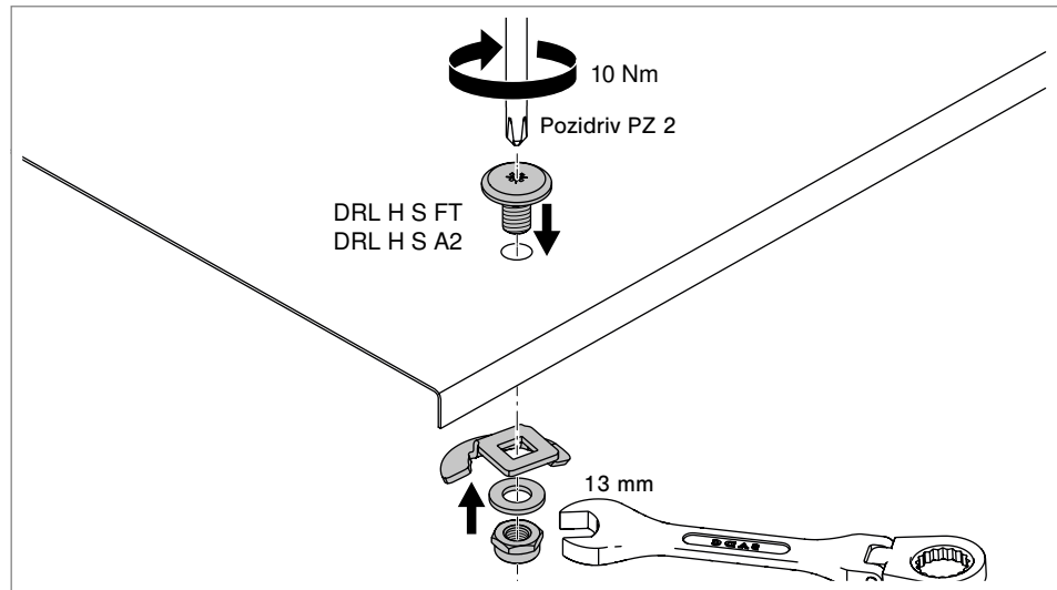
Figura 86: Aparafusar o ferrolho
