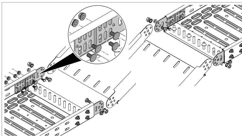
Figura 70: Montar as uniões articuladas nos caminhos de cabos em chapa
