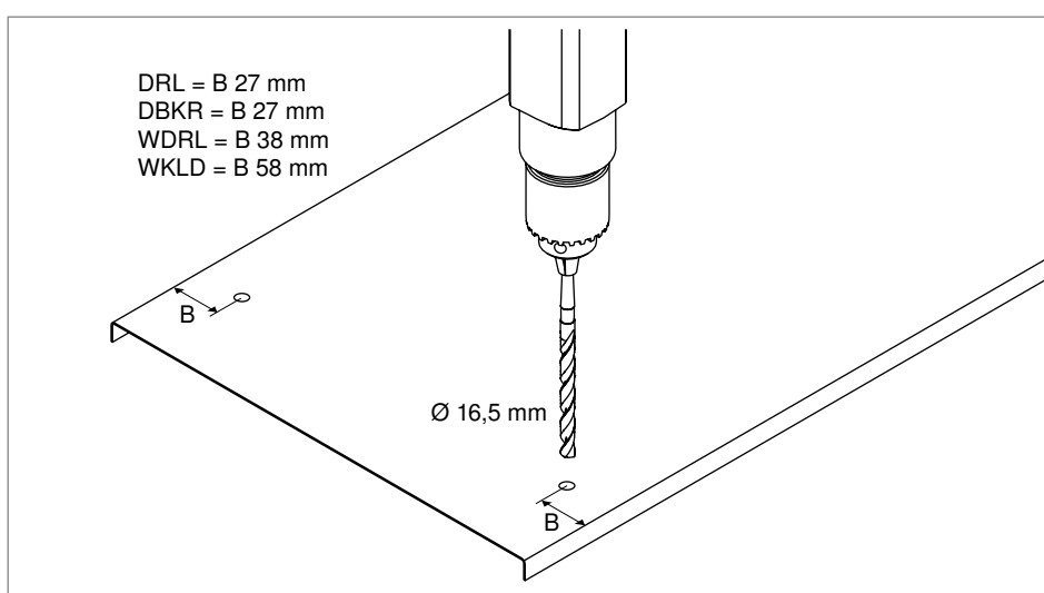
Figura 85: Pré-furar a tampa
