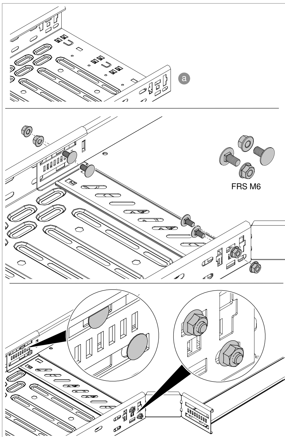
Figura 47: Fixar o acessório com parafusos (extremidade do caminho de cabos a)
