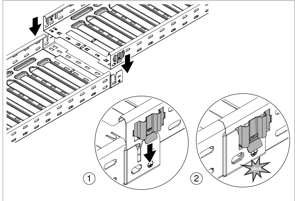
Figura 18: Ligação de encaixe Magic com elemento de mola
