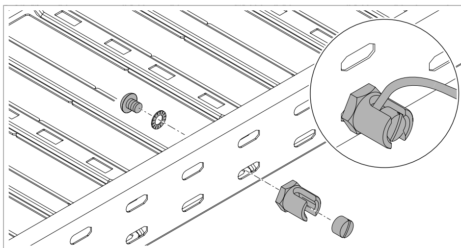
Figura 81: Montar o borne de terra
