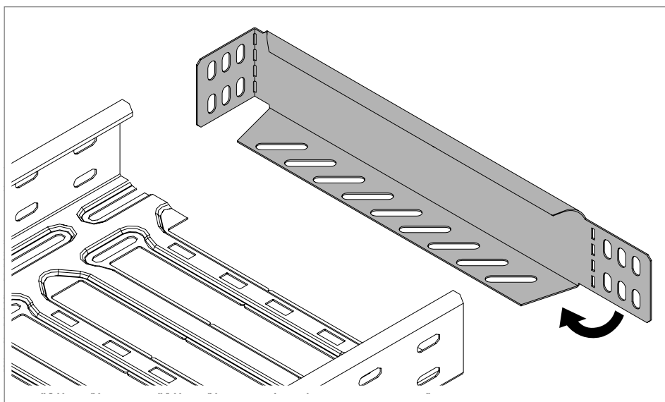
Figura 75: Dobrar a patilha
