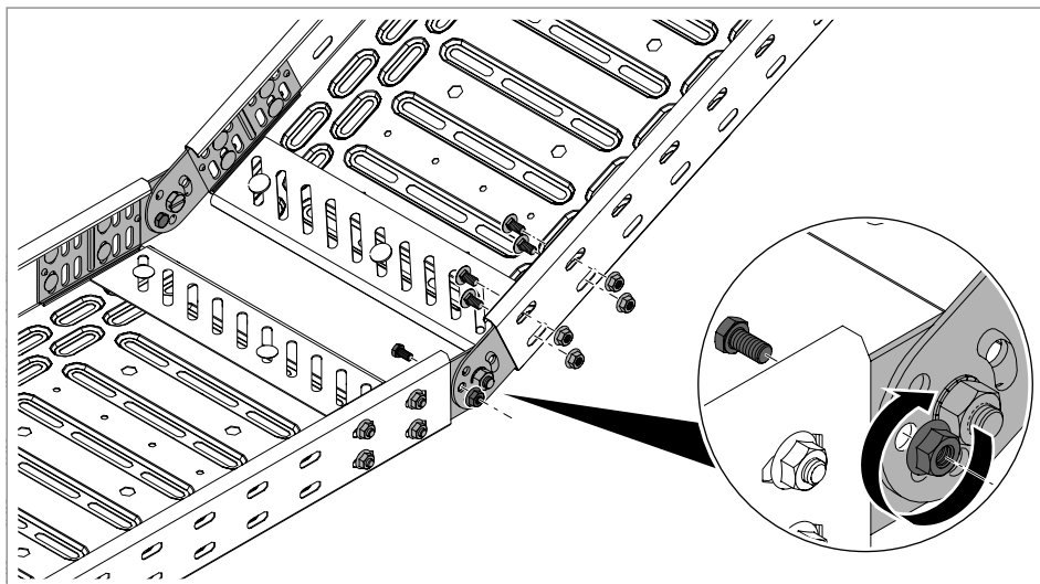
Figura 41: Apertar o parafuso de fixação
