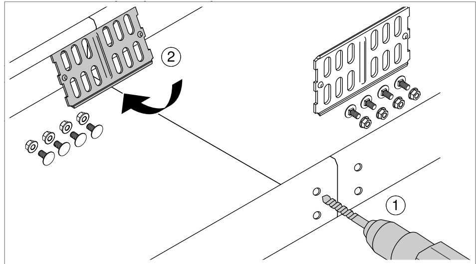
Figura 24: Introduzir as uniões retas RLVK
