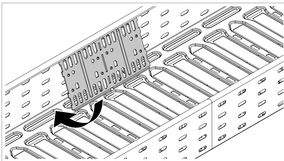
Figura 27: Introduzir as uniões RLVL
