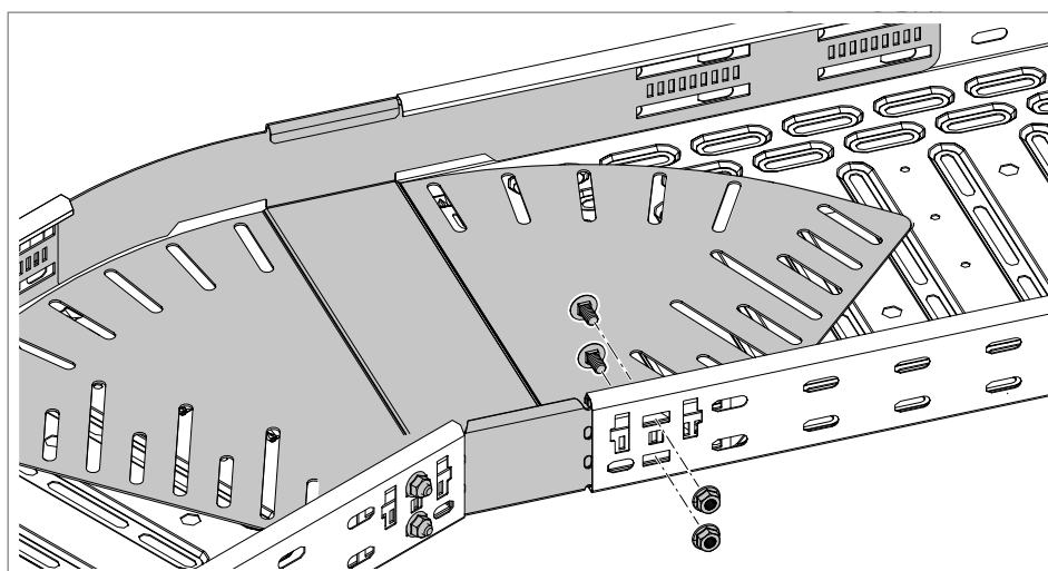
Figura 63: Fixar o segundo caminho de cabos ao ângulo
