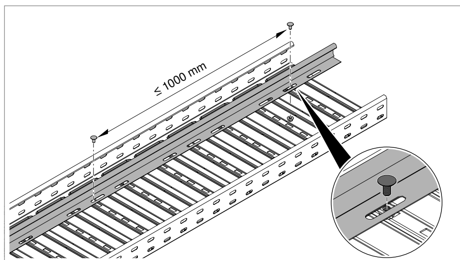
Figura 77: Aparafusar o separador
