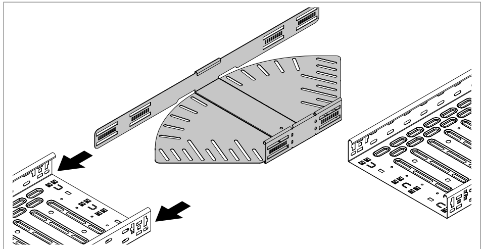
Figura 59: Inserir o ângulo variável
