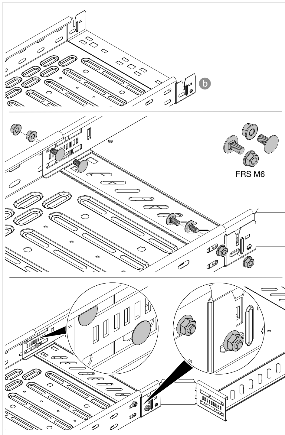
Figura 48: Fixar o acessório com parafusos (extremidade do caminho de cabos b)
