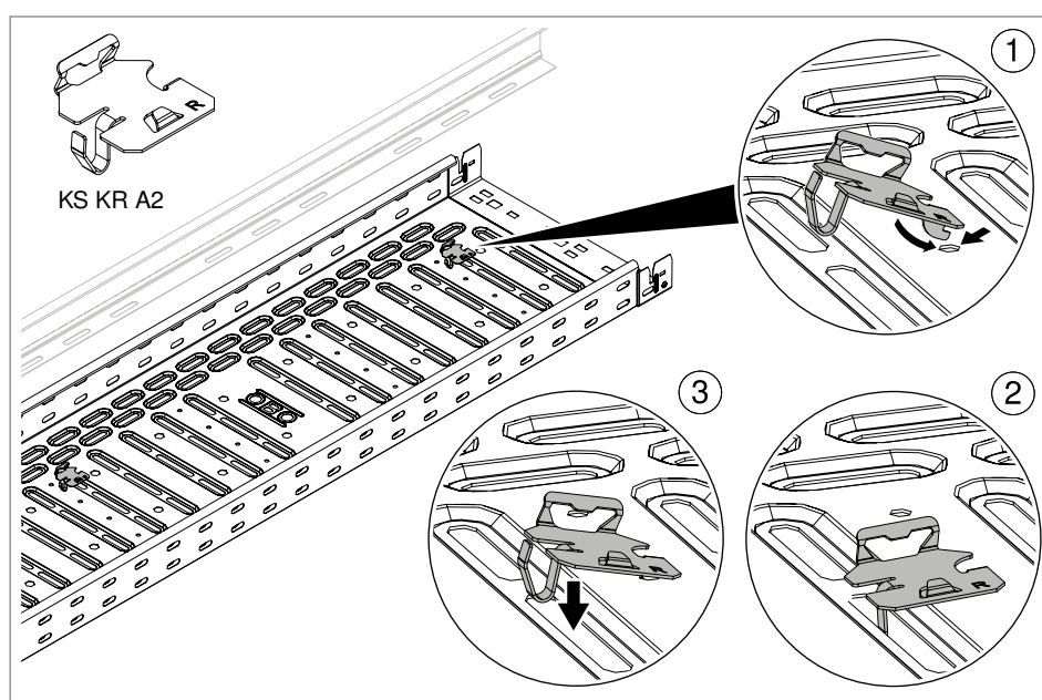
Figura 78: Inserir o fixador para separador
