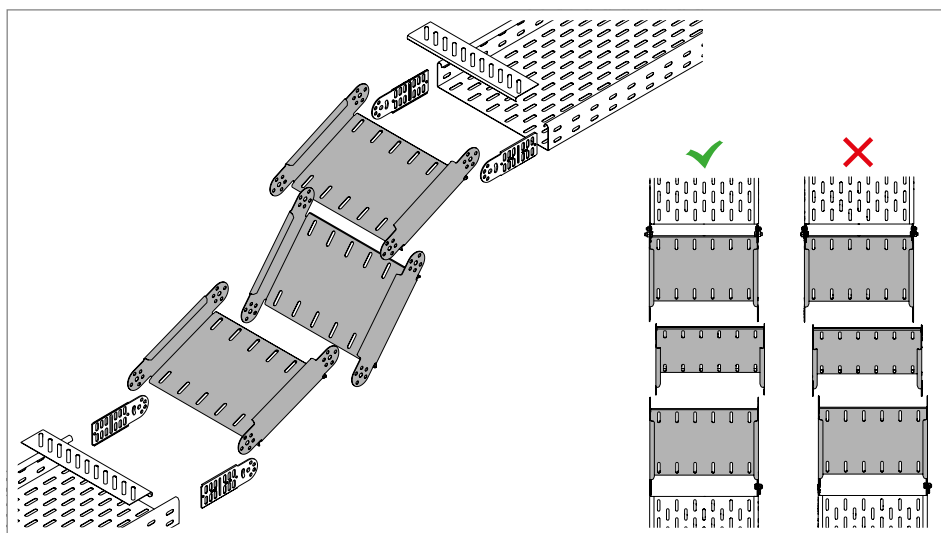
Figura 68: Elemento do ângulo regulável com uniões articuladas e placa de fundo
