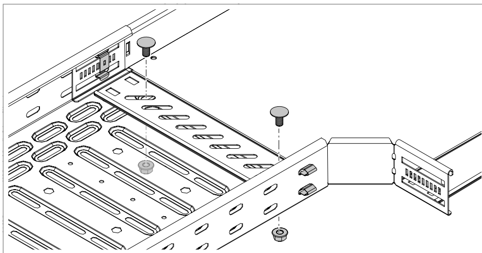
Figura 51: Aparafusar a régua tapa juntas
