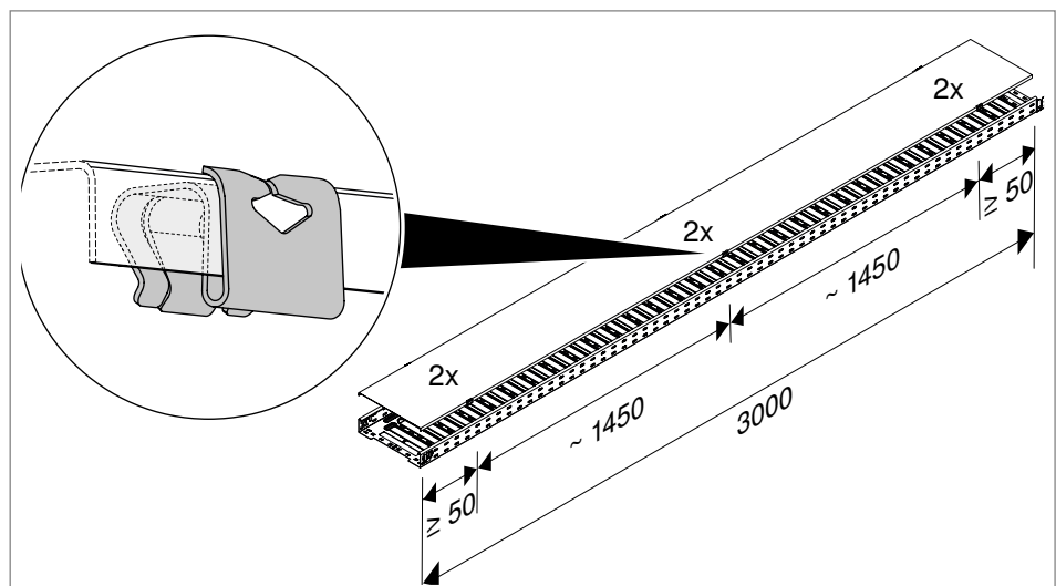
Figura 83: Distribuição do número necessário de grampos para tampa
